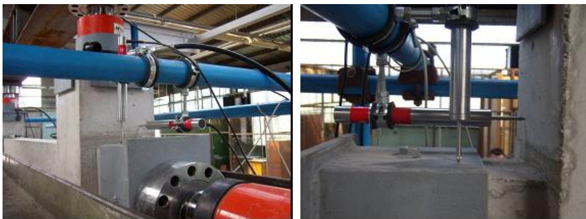
Slika 4.14 Prikaz horizontalnih i vertikalnih LVDT_a za mjerenje pomaka
