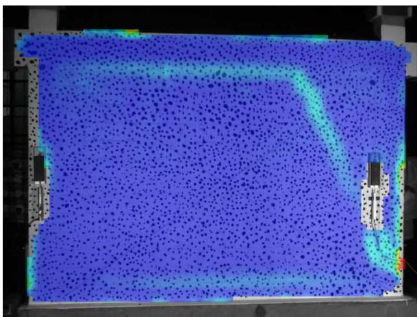
c) Prva značajna pukotina pri pozitivnom smjeru opterećenja (ARAMIS)
