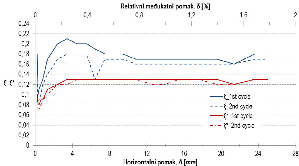
Slika 6.57 Ovisnost prigušenja ispitanog uzorka O1_cvm o horizontalnom pomaku
