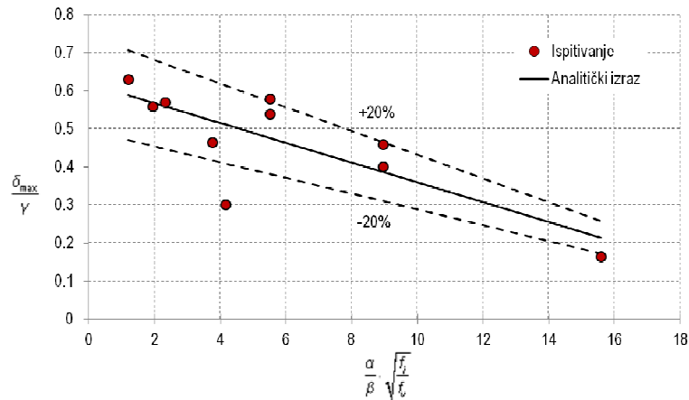
Slika 7.23 Usporedba eksperimentalnih i analitički procijenjenih vrijednosti \delta_{max}
