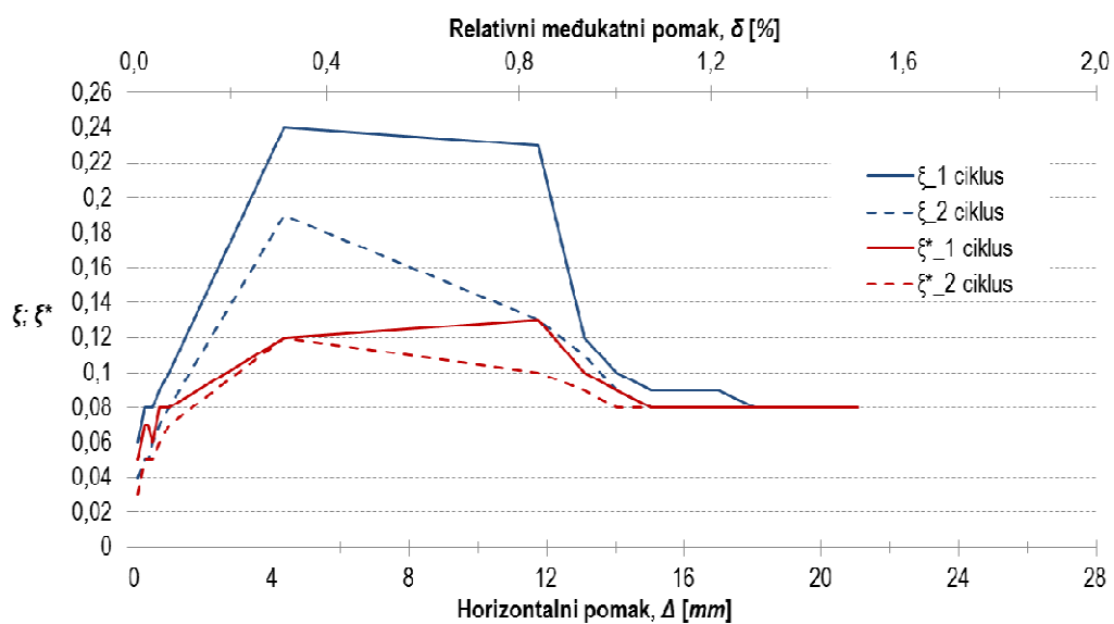
Slika 6.47 Prigušenje ispitnog uzorka O1_bvm u ovisnosti o načinu izračuna apsorbirane energije
