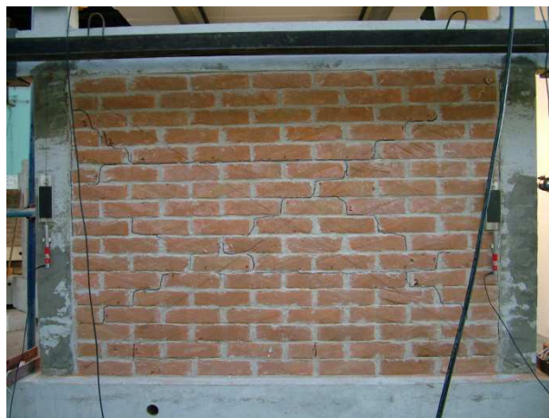
Slika 6.59 Prve značajne pukotine u ispuni ispitnog uzorka O1_cvm
