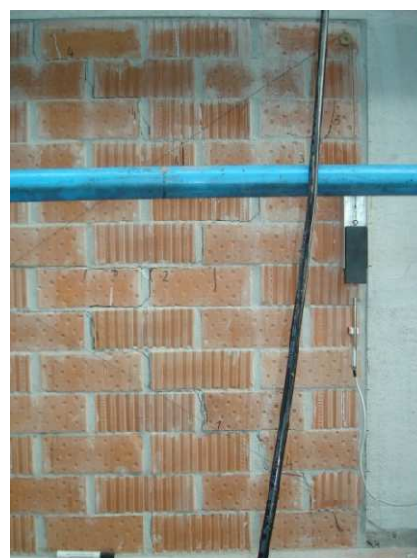
Slika 6.50 Prikaz prvih pukotina ispitnog uzorka O1_bvm
