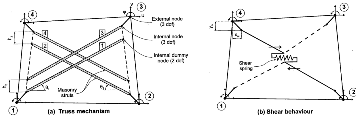
Slika 2.2 Ciklički model ponašanja zidanog ispuna pri a) tlačnom i b) posmičnom opterećenju [13]
