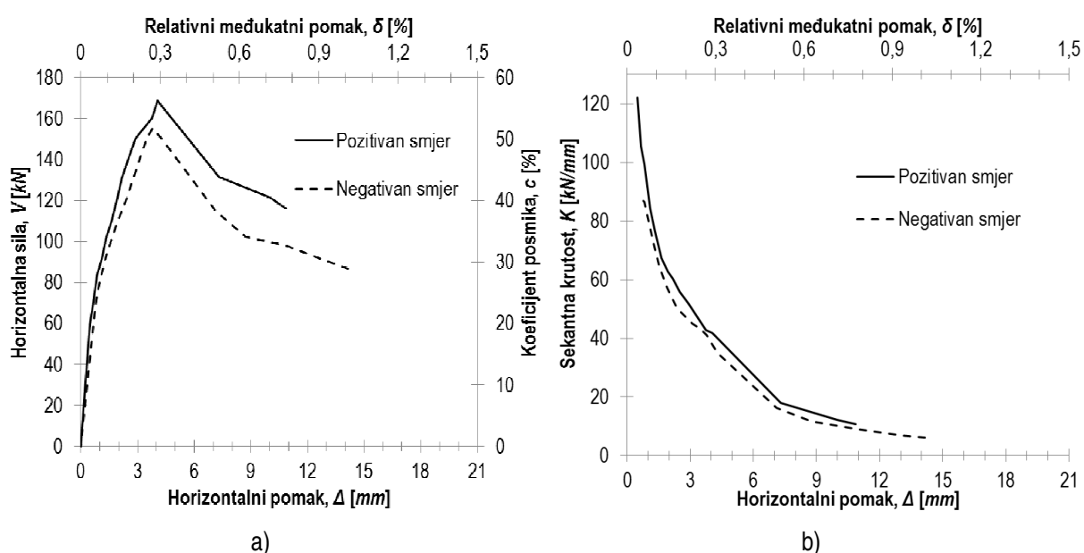
Slika 6.20 Prikaz primarnih krivulja odgovora i sekantne krutosti, u ovisnosti o pomaku, pri pozitivnom i negativnom smjeru opterećenja ispitnog uzorka O1_bpm
