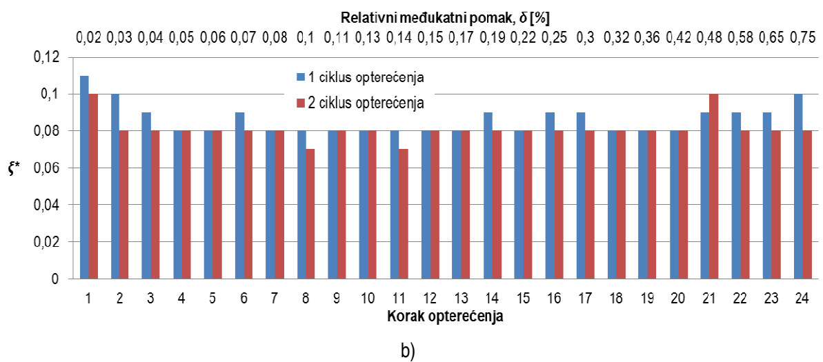
Slika 6.105 Prigušenje ispitnog uzorka O3_cpm u ovisnosti o načinu izračunu apsorbirane energije
