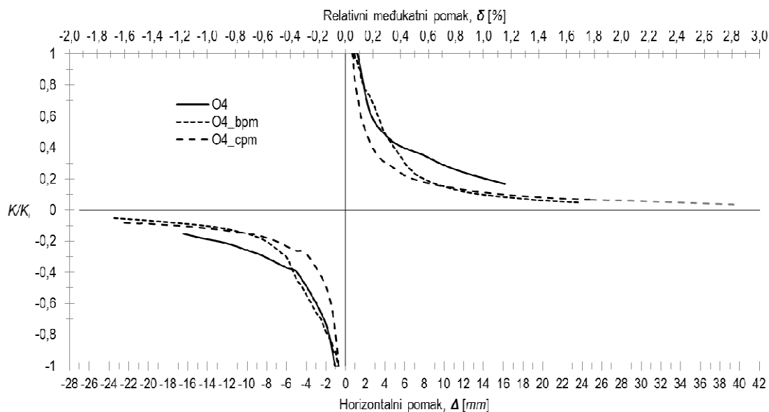
Slika 6.158 Prikaz degradacije sekantne krutosti ispitnih uzoraka skupine O4 u ovisnosti o horizontalnom pomaku
