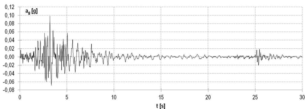
Slika B1.5 Prikaz akceleroograma, spektra energije i idealiziranih spektara ubrzanja i pomaka za zapis potresa Spitak_y.
