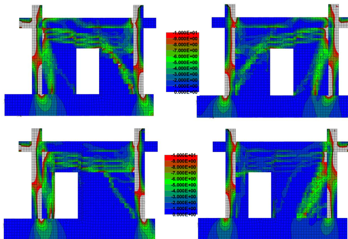
Slika 6.12. Raspodjela glavnih tlačnih naprezanja pred slom za IDR=1,0 % modela tip (IV/11) gore i tip (IV/12) dolje
