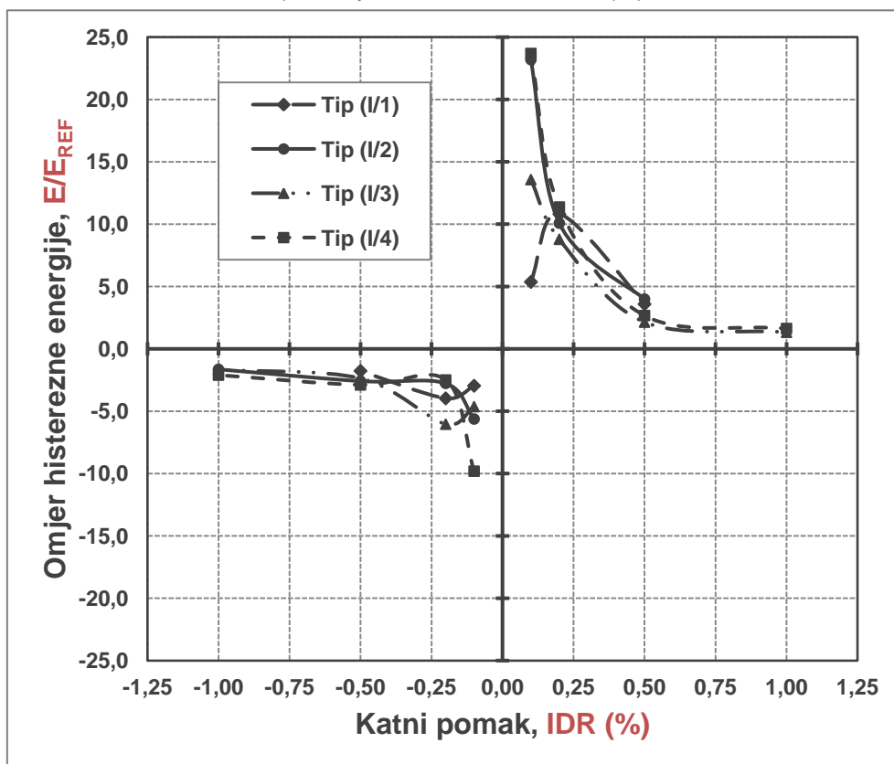
Slika 4.7. Histerzna energija uzoraka grupe I, E (kNm) i omjer energije, E/E_{REF} u odnosu na energiju praznog okvira pri jednakom katnom pomaku, IDR (%)
