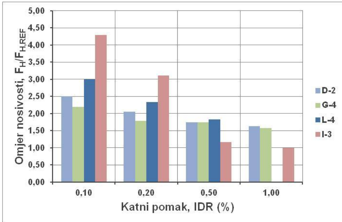
Slika 8.5. Usporedba faktora utjecaja na nosivost za zidane ispunne odnosa stranica H/L_1=0,93 u odnosu na katne pomake IDR (%)
