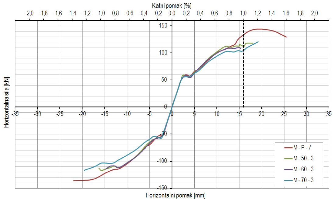
Slika 6.36 - Nosivost čeličnih okvira s kombiniranim ispunom – varijacije oslabljenja porobetonских elemenata – P, 50, 60, 70; čvrstoće 3 i 7
