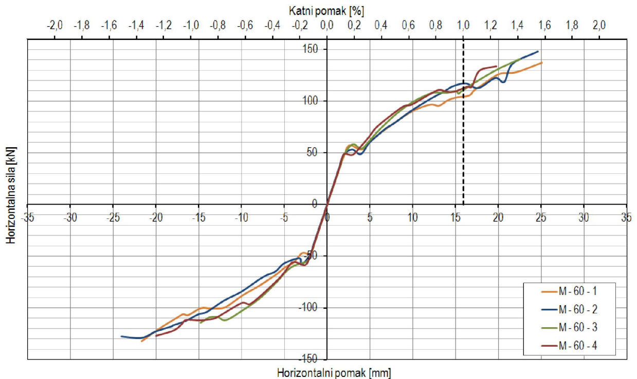
Slika 6.37 - Nosivost čeličnih okvira s kombiniranim ispunom – varijacije kvalitete porobetonских elemenata – 1, 2, 3, 4; debljina oslabljenja 60
