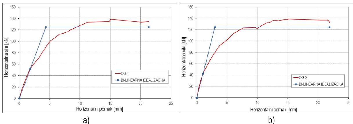
Slika 8.2 – Eksperimentalna i idealizirana bi-linearne anvelope nosivosti: a) uzorak OG-1, b) uzorak OG-2
