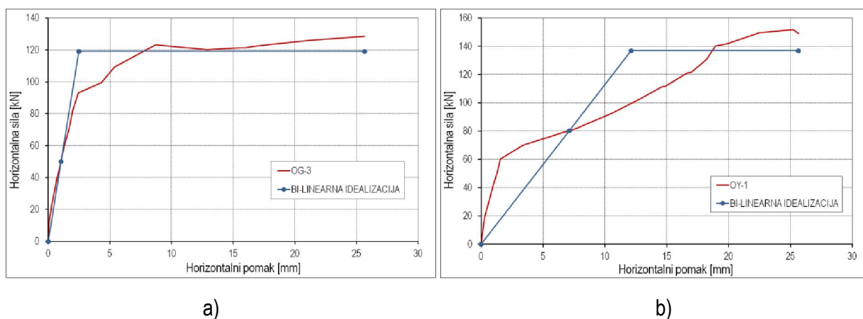
Slika 8.3 – Eksperimentalna i idealizirana bi-linearne anvelope nosivosti: a) uzorak OG-3, b) uzorak OY-1
