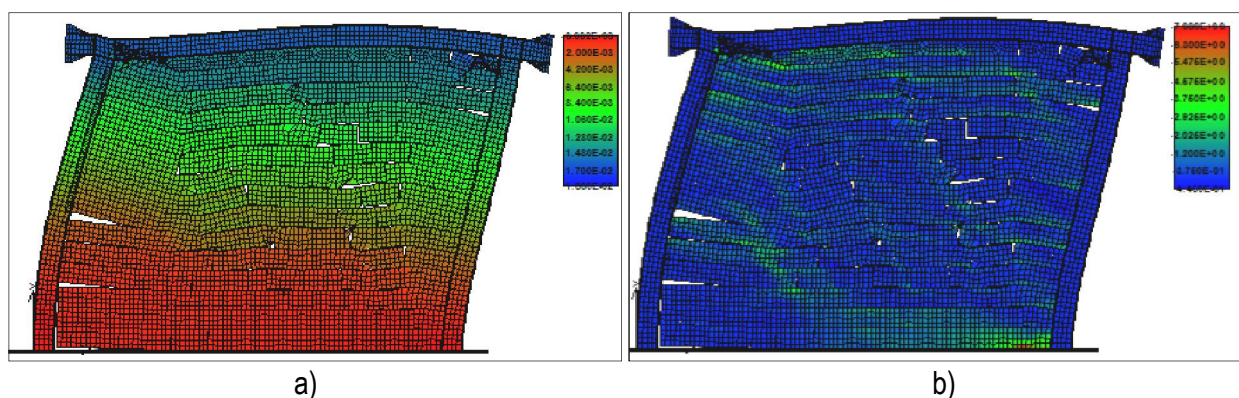
Slika 5.66 – Horizontalni pomaci čeličnog okvira (a) i normalna naprezanja (b) u glinenom zidanim ispunu pri međukatnom pomaku od 1,0 %
