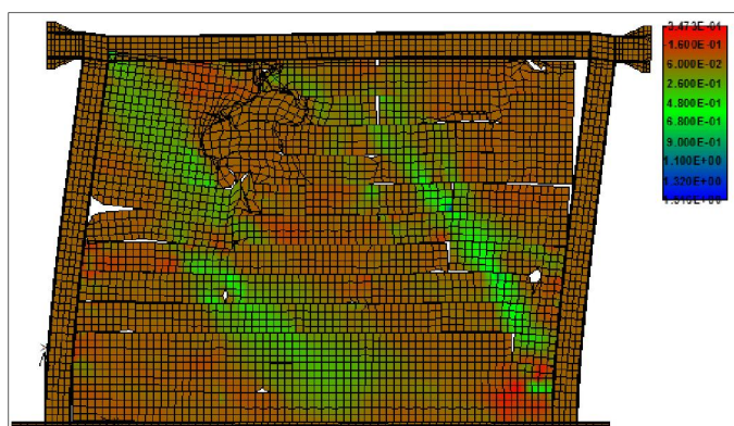
Slika 5.87 – Posmična napreznja u porobetonskom ispunu pri slomu
