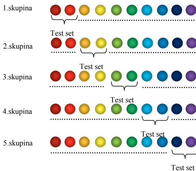
Slika 26. 5-fold unakrsna validacija (..... – set za treniranje)
