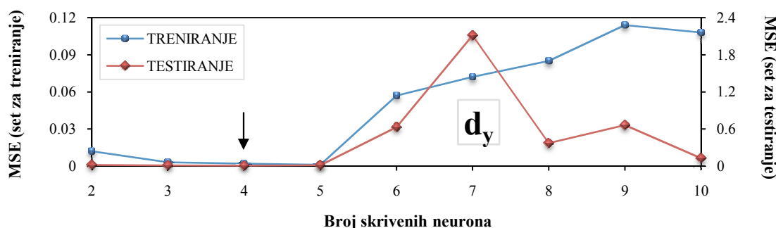
Slika 31. Srednja kvadratna pogreška na setu za treniranje i testiranje u ovisnosti o broju skrivenih neurona za pomak u području popuštanja
