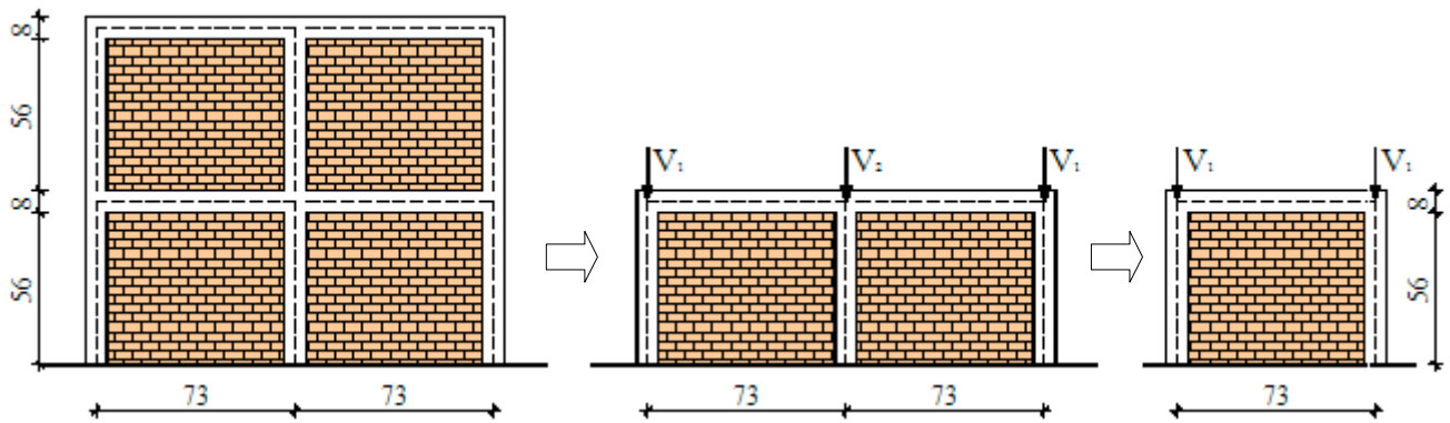
Slika 82. Model aproksimacije za višekatnu i višerasponsku građevinu IFS
