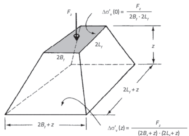
Slika 2. Približna raspodjela vertikalnog naprezanja ispod kvadratnog temelja, prema metodi 2:1 [31] (uredili autori)
