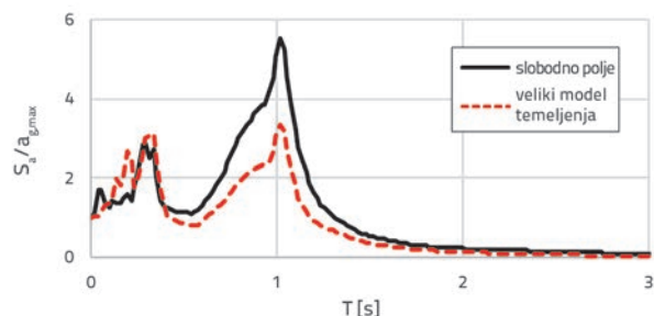
Slika 8. Spektri odziva dobiveni iz eksperimenta u centrifugi na Sveučilištu u Cambridgu za slobodno polje (puna crna linija) i ispod temelja teškog modela (isprekidana crvena linija)
