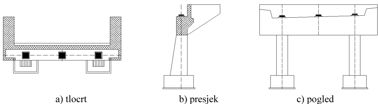
Slika 6.5 – Olakšani upornjak
