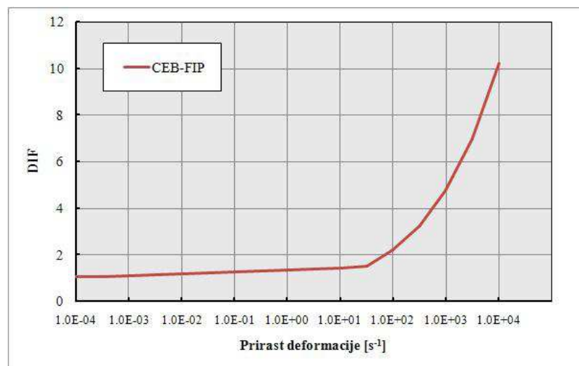
Slika 7.10 – DIF za tlačnu čvrstoću betona
