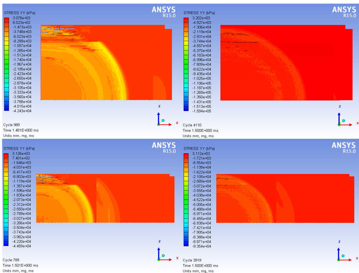
Slika 9.11 – Naprezanje donje plohe rasponske konstrukcije u t=1,5 ms
