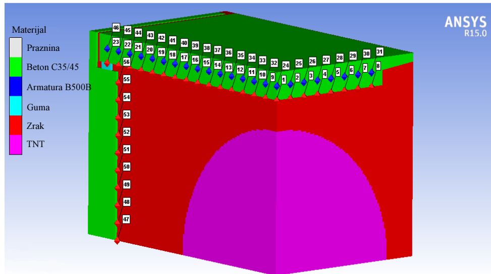
Slika 9.1 – Raspored mjernih točaka na nadvožnjaku Tip 1
