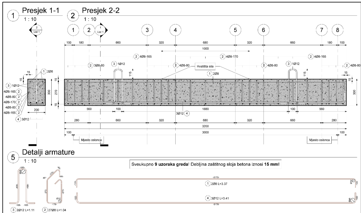
Slika 7.5 AB grede - armaturni nacrti i specifikacija količina armaturnih šipki – dvodimenzionalni prikaz
