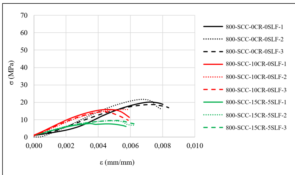
Slika 6.49 Odnos naprezanje-deformacija uzoraka izloženih visokoj temperaturi od 800 °C
