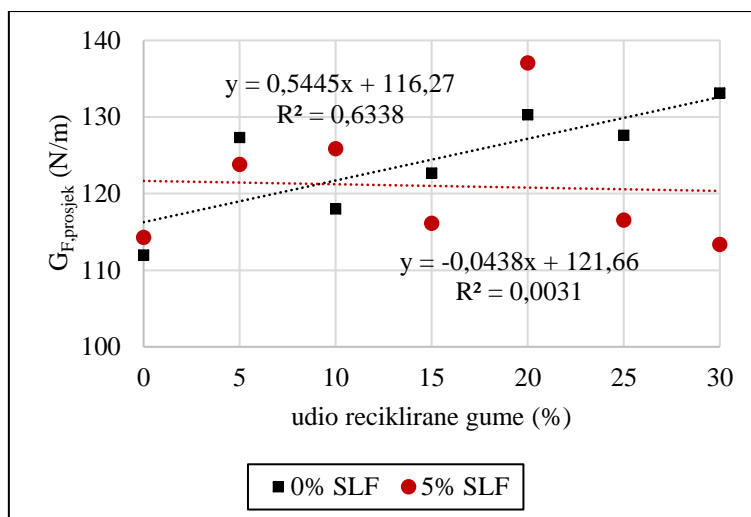
Slika 5.24 Energija loma ispitanih uzoraka samozbijajućeg betona kada je CMOD = 0,5 mm
