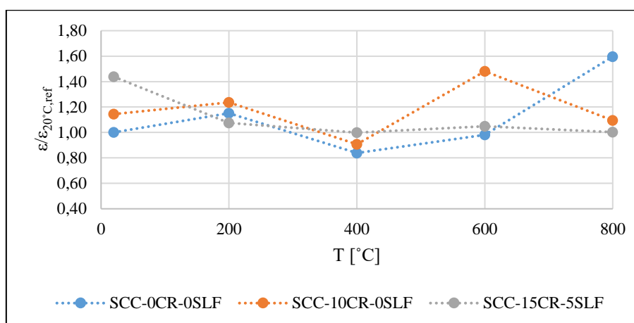
Slika 6.44 Normalizirane vrijednosti deformacije pri maksimalnom naprezanju u odnosu na vrijednost deformacije pri maksimalnom naprezanju referentne mješavine pri T = 20 °C
