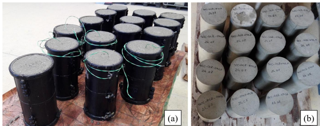
Slika 6.10 Cilindrični betonski uzorci u svježem stanju (a) i očvrnulom stanju (b)
