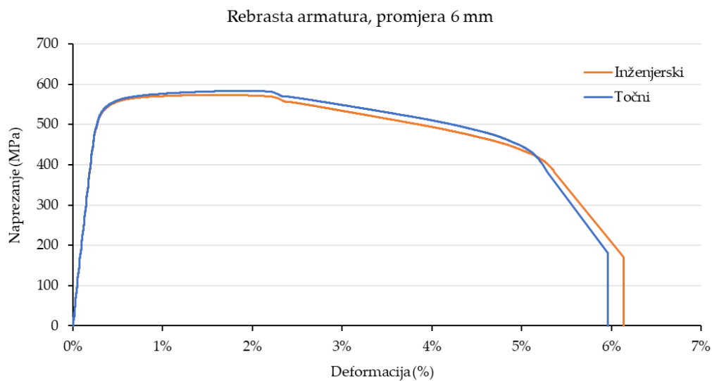
Slika 7.8. Grafički prikaz prosječnih rezultata ispitivanja točnog i inženjerskog naprezanja i deformacije poprečne armature
