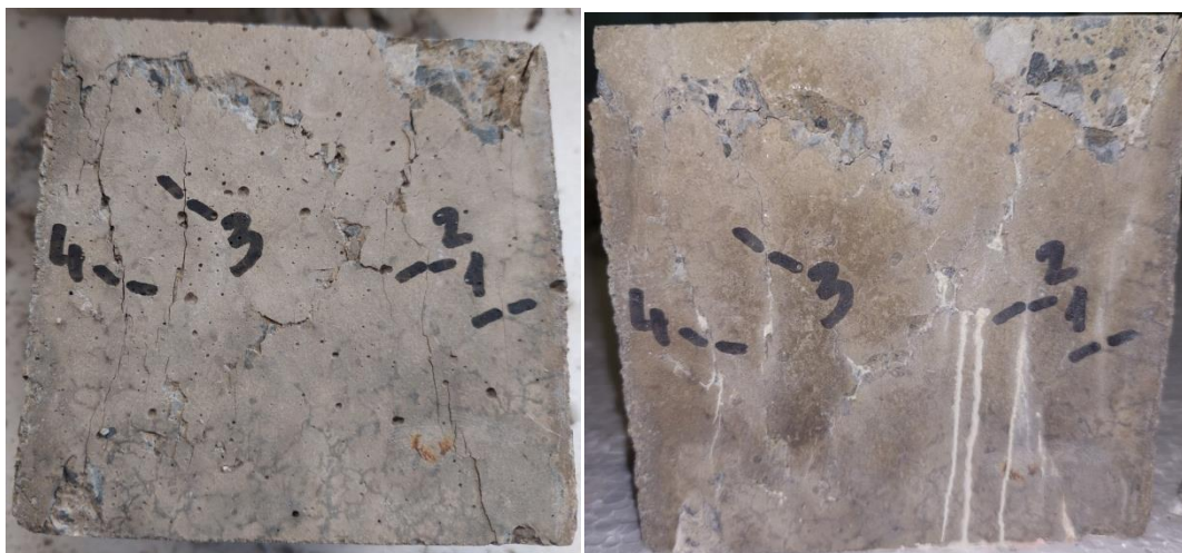
Slika 6.77. Mješavina M6 bez smrzavanja (lijevo – prije samocijeljenja, desno - nakon samocijeljenja)
