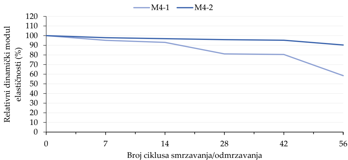
Prilog 40. Pojedinačni rezultati ispitivanja unutarnjih oštećenja uslijed ciklusa smrzavanja i odmrzavanja bez soli mješavine M4
