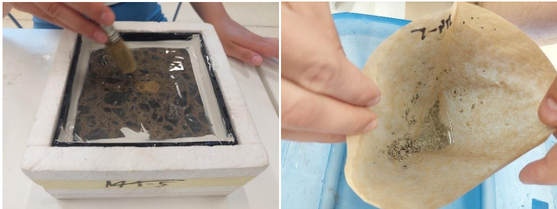
Slika 6.28. Ispitivanje otpornosti betona na cikluse smrzavanja/odmrzavanja-ljuštenje
