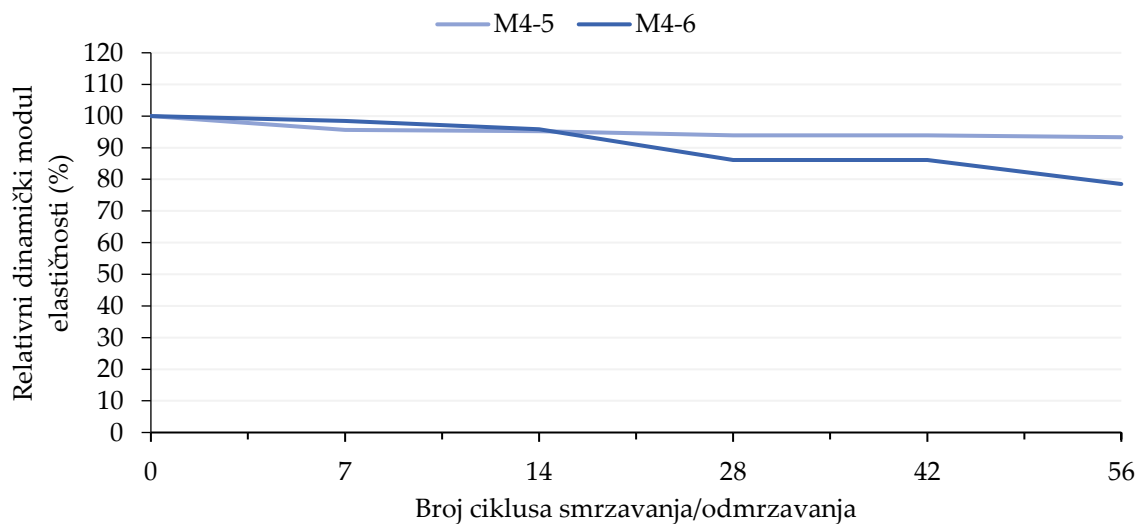
Prilog 41. Pojedinačni rezultati ispitivanja unutarnjih oštećenja uslijed ciklusa smrzavanja i odmrzavanja sa soli mješavine M4
