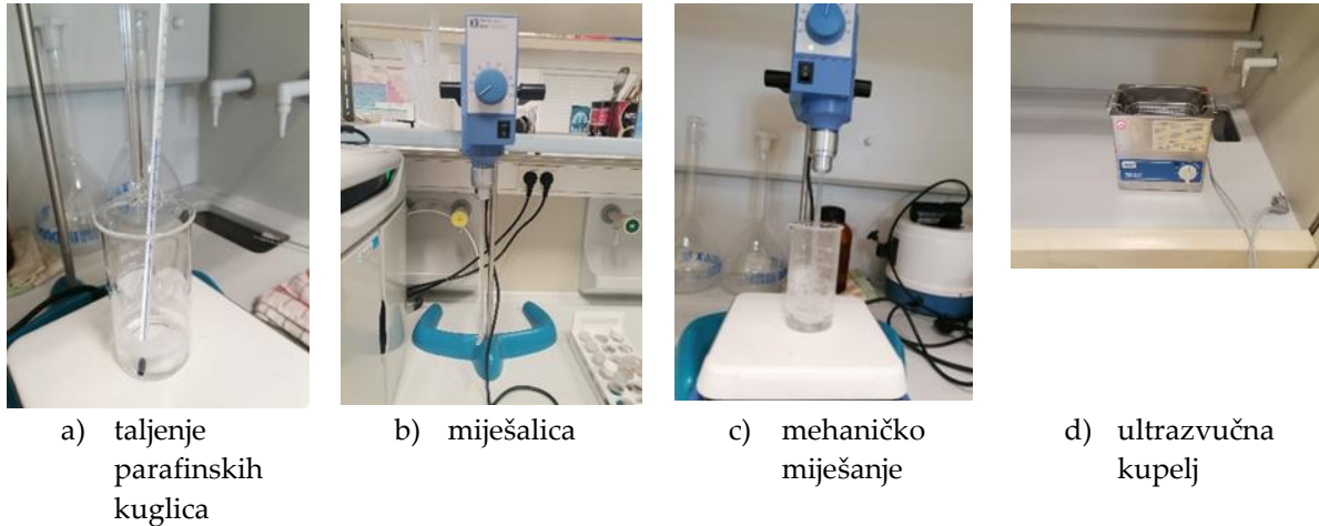
Slika 6.7. Postupak proizvodnje mikrokapsula
