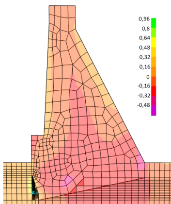
Slika 12. Raspodjela normalnih napreznosti po tijelu brane za kritičan slučaj – potres u Albaniji, stijena pješčenjak, 2. kombinacija opterećenja
