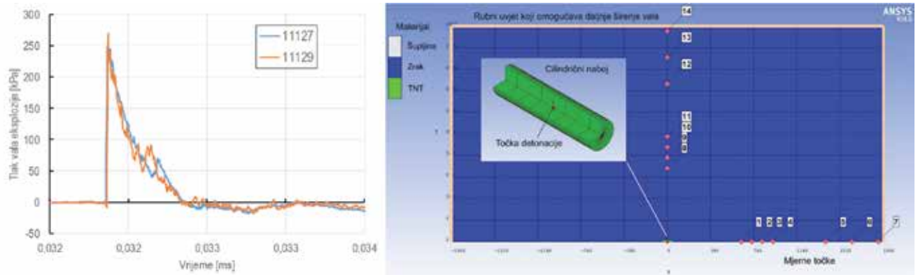
Dijagram mjerenoga tlaka za bočne senzore (lijevo) i numerički model eksperimenta (desno)
