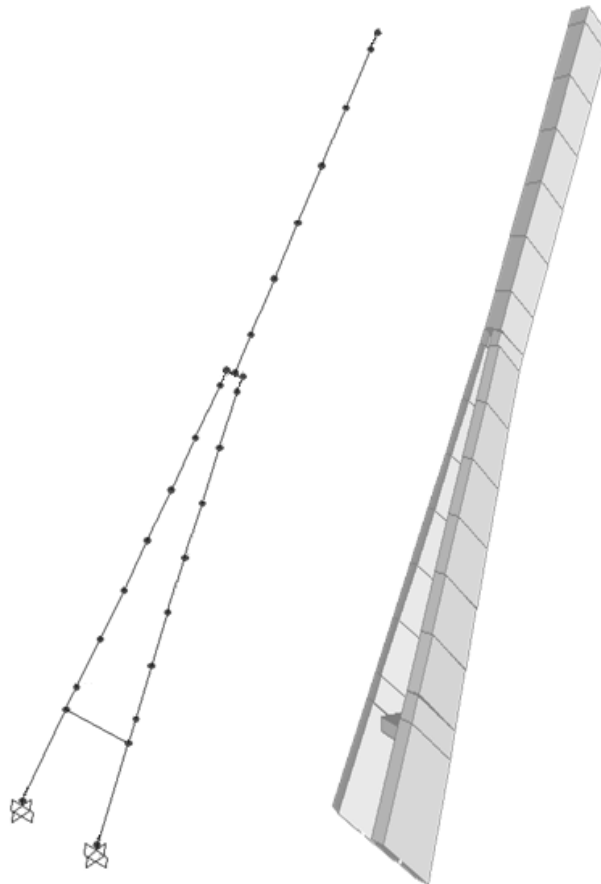
Slika 14 – Model pilona
