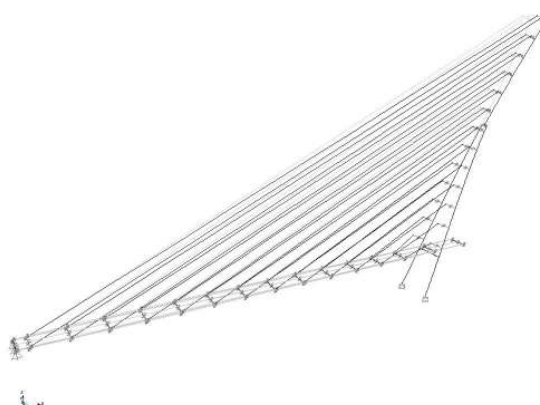
Slika 16 – Vlastiti oblik 2.
