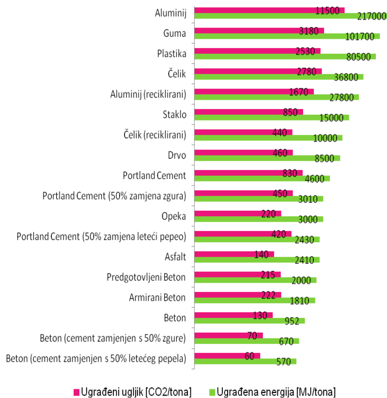
Slika 2 – Ugrađena energija (EE) i ugrađeni ugljik (EC) najčešćih građevinskih materijala [2]
