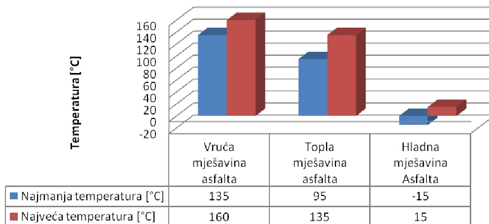
Slika 6 – Temperaturni raspon pri nanošenju asfalta [16, 17]
