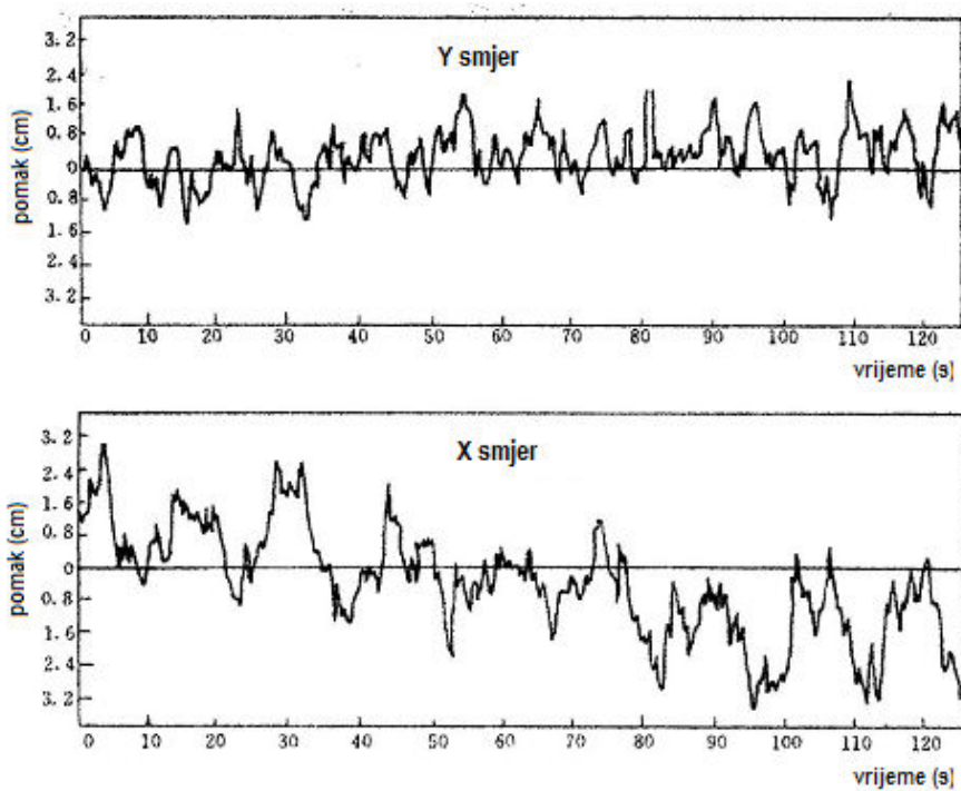
Slika 8 – Dijagram pomak-vrijeme
