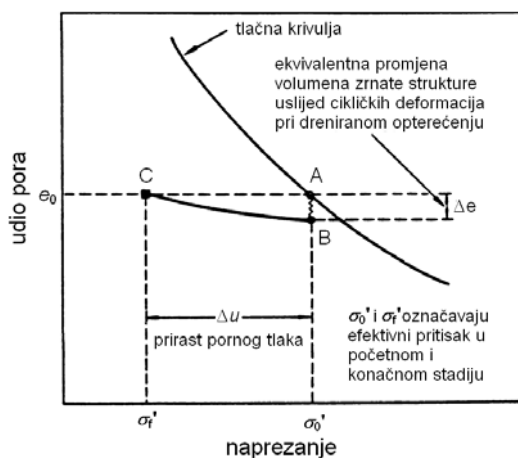
Slika 2 - Porast pornog tlaka pri cikličkom naprezanju [2] (sliku prilagodili autori)
