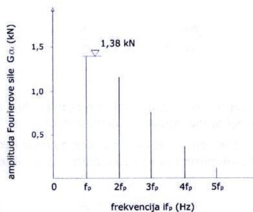
Slika 6 - Diskretni Fourierov spektar za dinamičku silu prikazanu na slici 5 [2]
