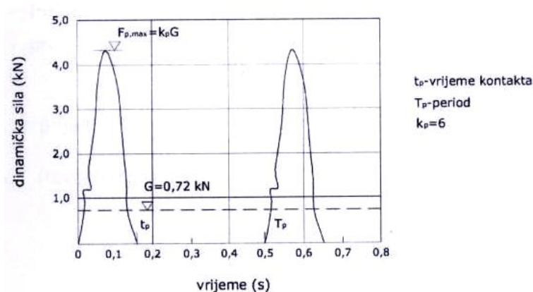
Slika 5 - Primjer funkcije dinamičke sile zbog skakanja na mjestu s obje noge istovremeno, f = 2 Hz [2]
