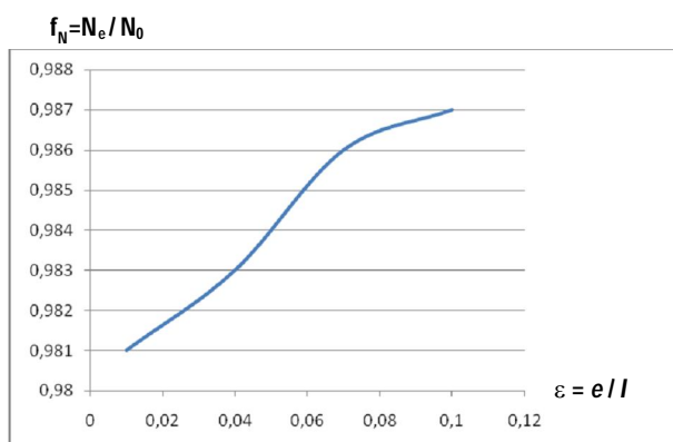
Slika 12 – Promjenjivost uzdužne sile u tlačnom pojasu – ekscentricitet u oba pojasa
