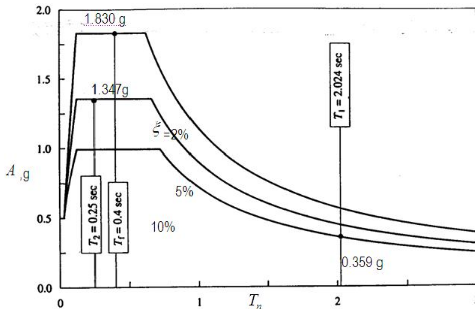
Slika 8 - Projektni spekatar i ordinate spektra za izoliranu građevinu i građevinu s fiksnom bazom
