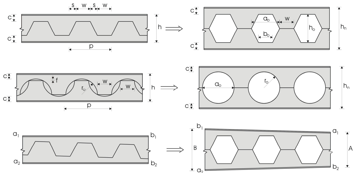
Slika 1 – Sačasti nosači
