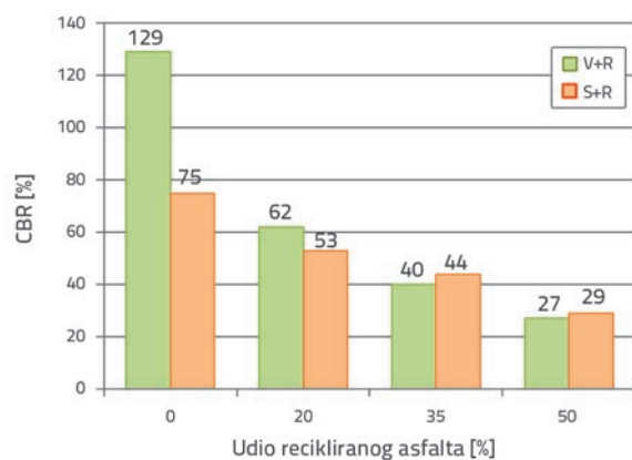
Slika 10. Vrijednost CBR-a u ovisnosti o udjelu recikliranog asfalta
