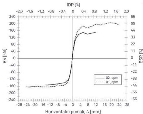
Slika 14. Primarne krivulje odgovora uzorka O1 cpm i O2 cpm
