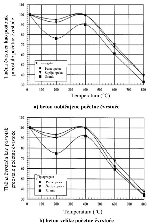
Slika 4. Redukcija tlačne čvrstoće betona pri izlaganju visokim temperaturama [14]
