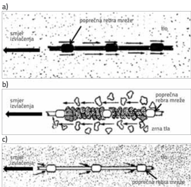
Slika 6. Mehanizmi interakcije tla i geomreže: a) trenje na kontaktu s mrežom; b) trenje po česticama tla uklještenog u otvore mreže; c) djelovanje pasivnog otpora tla na poprečna rebra mreže [36]
