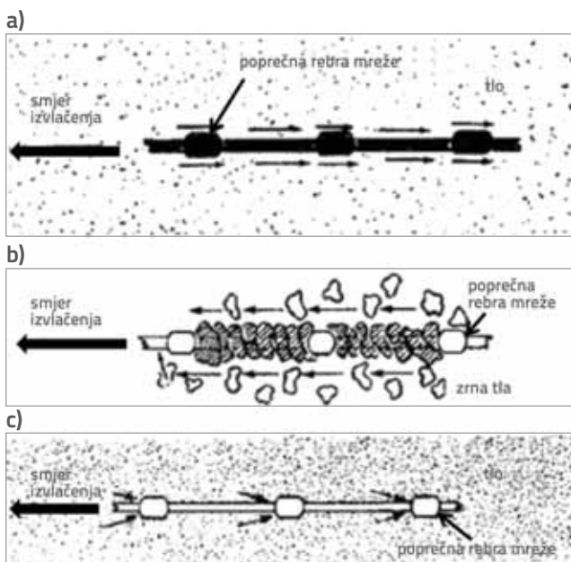
Slika 6. Mehanički interakcije tla i geomreže: a) trenje na kontaktu s mrežom; b) trenje po česticama tla uklještenog u otvore mreže; c) djelovanje pasivnog otpora tla na poprečna rebra mreže [36]
