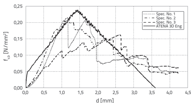
Slika 7. Dijagram odnosa pomaka i posmične čvrstoće зида за смјер хоризонталних слјубница
