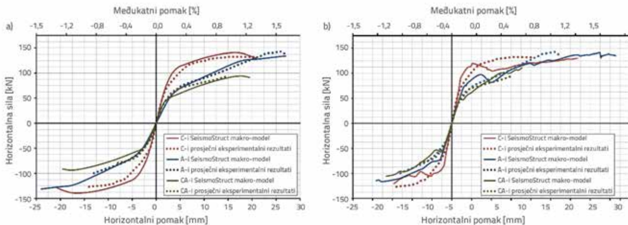
Slika 10. Primarne krivulje dobivene pomoću: a) makromodela (Seismostruct); b) mikromodela (Atena 2D)
