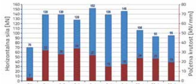
Slika 4. Nosivosti i početne krutosti čeličnog okvira (BF) i okvira s ispunom od šupljih glinenih blokova (C- i ), porobetonskih blokova (A- i ) i s kombiniranom ispunom (CA- i )
