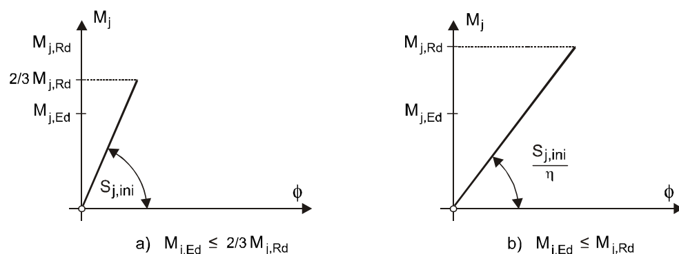
Slika 1. Rotacijska krutost priključaka za proračune po teoriji elastičnosti
