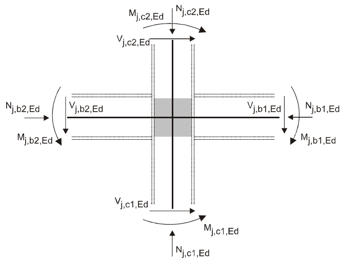
Sile i momenti u presjecištu težišnih linija spojenih elemenata
