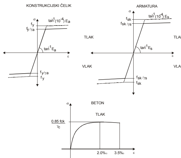
Slika 8. Proračunski radni dijagrami materijala primijenjeni pri proračunu
