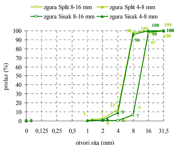
Slika 2. Krivulje prosijavanja zgure iz Splita, frakcije 4-8 i 8-16 mm
