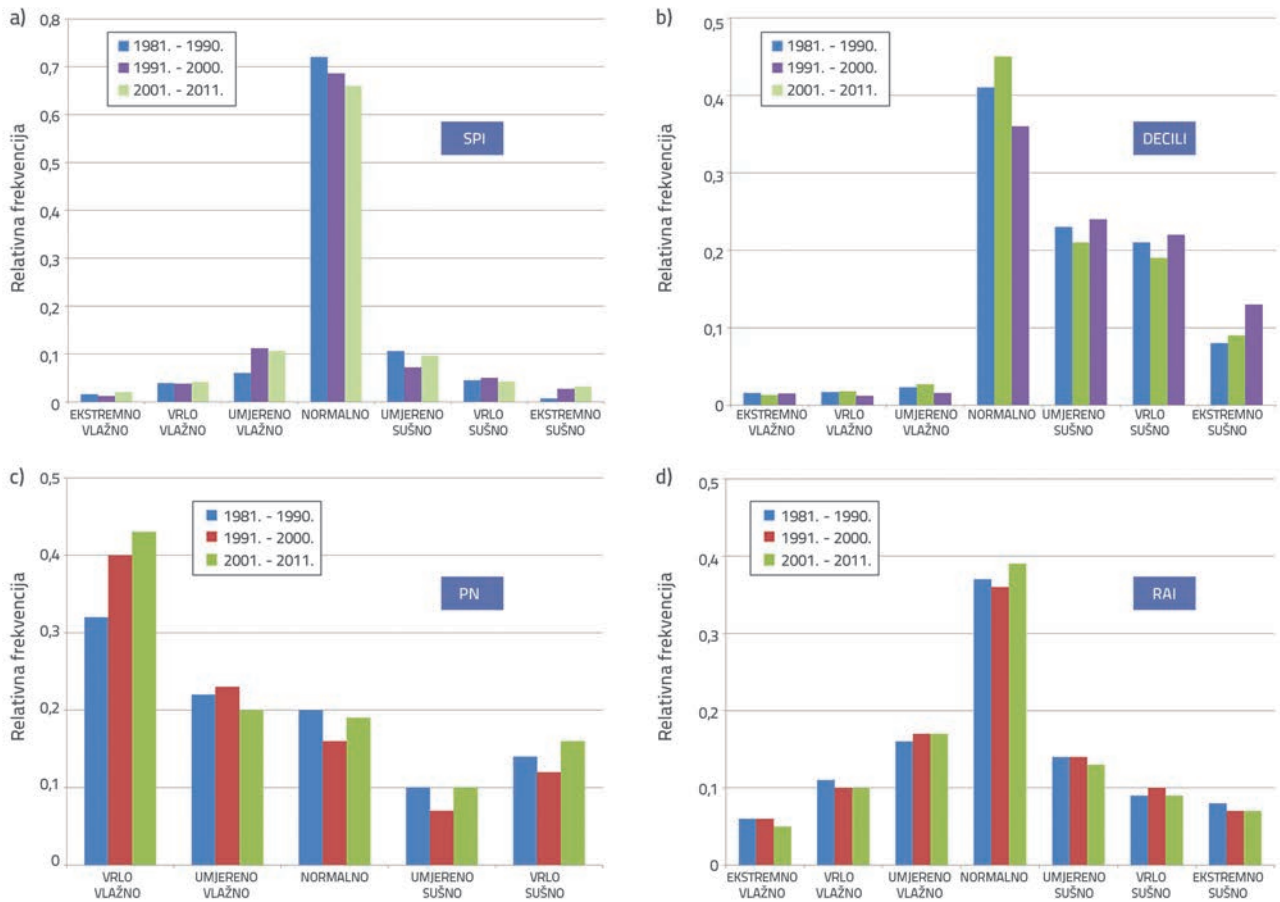
Slika 2. Relativna frekvencija vlažnih i sušnih godina prema: a) SPI; b) Decilima; c) PN; d) RAI. Relativne frekvencije su prikazane za svako od podrazdoblja (1981.-1990., 1991.-2000. i 2001.-2011.)
