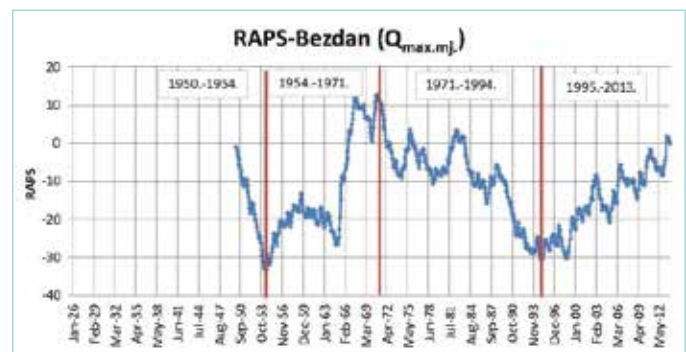
Slika 18. RAPS maksimalnih godišnjih protoka rijeke Dunav zabilježenih na postaji Bezdan u razdoblju od 1950. do 2013. god.
